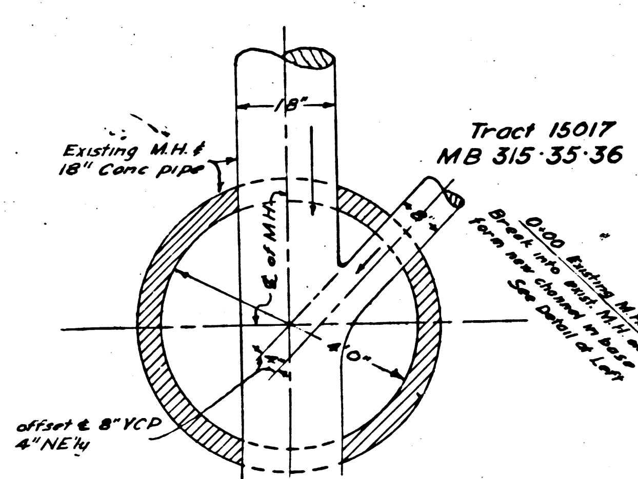
VICTORIA AVE, MANHOLE DETAIL SCALE: 6"=1'
