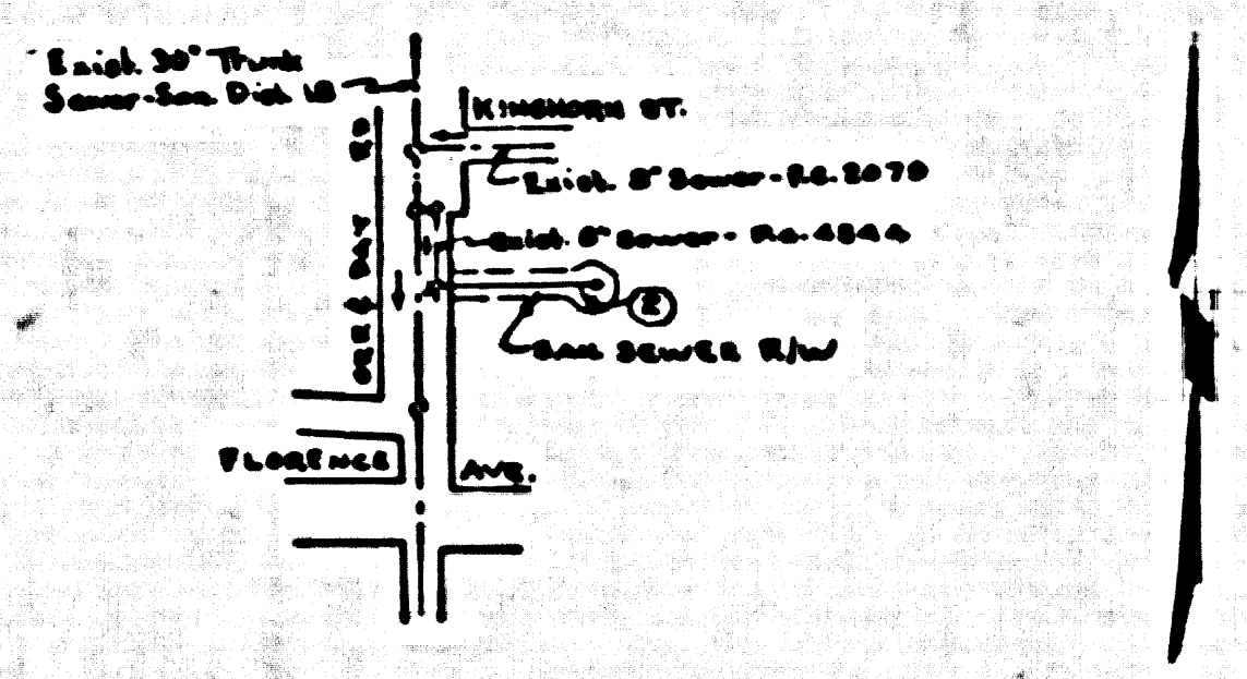
INDEX MAP RC 4664 SCALE: 1" = 600'
