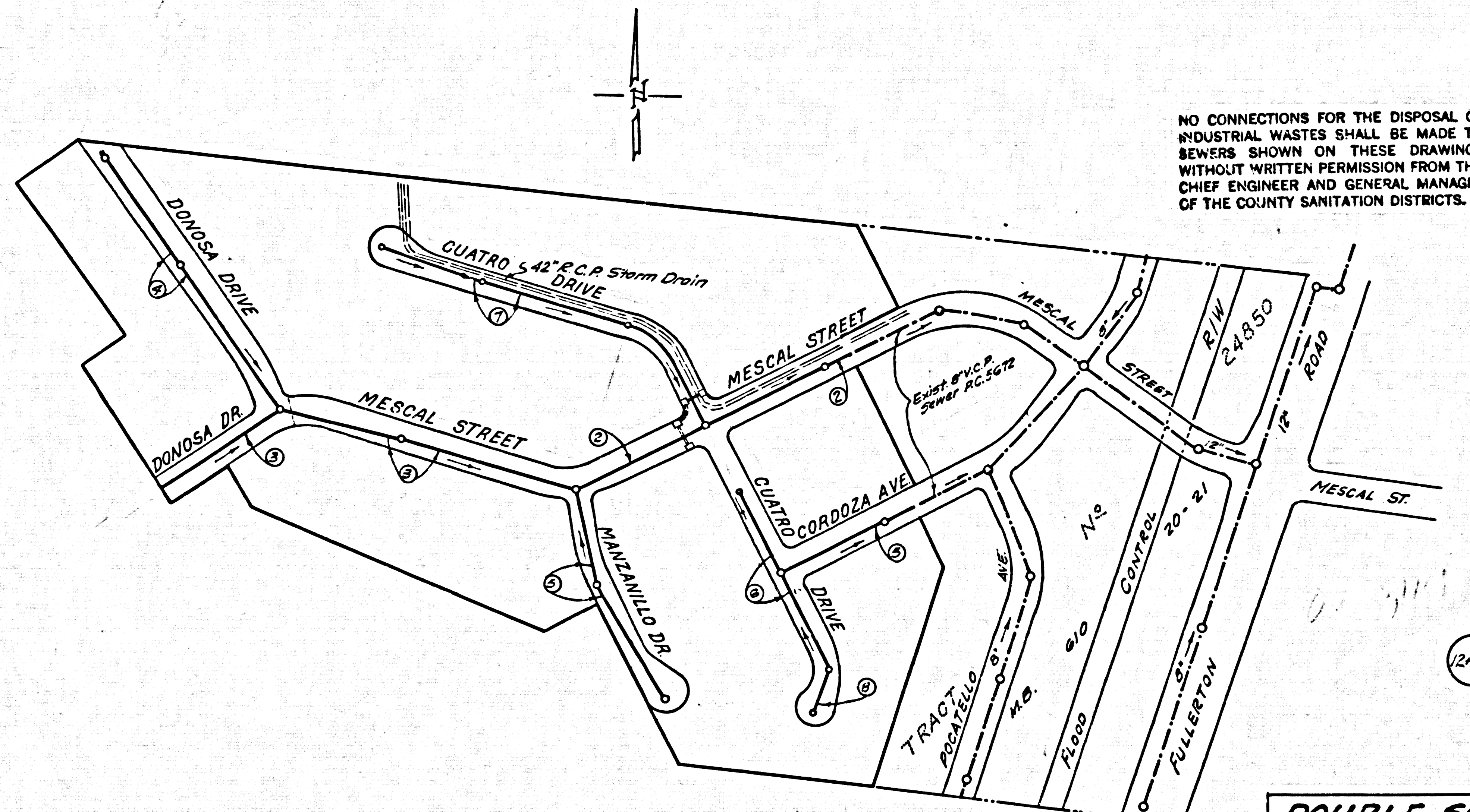
INDEX MAP Scale: 1"=200' P.C. 6015
