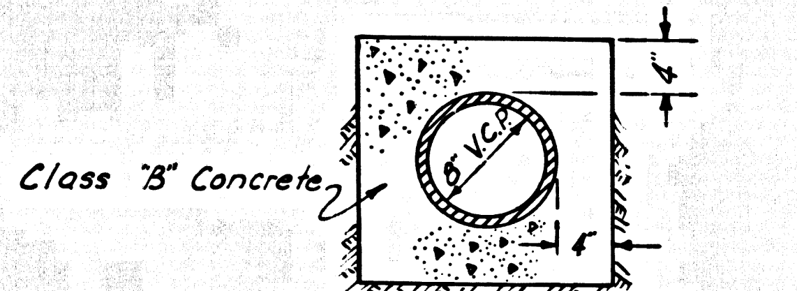
ENCASEMENT DETAIL SCALE: 1"=1'-0" Sta. 2+85 TO Sta. 5+23.57
