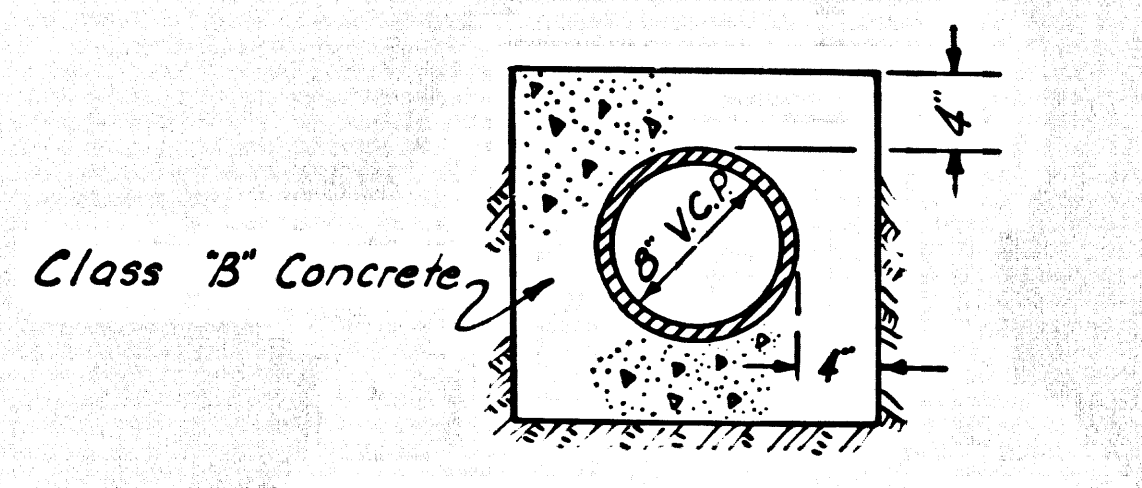
ENCASEMENT DETAIL SCALE: 1"=1'-0" Sta. 2+65 TO Sta. 5+23.57
