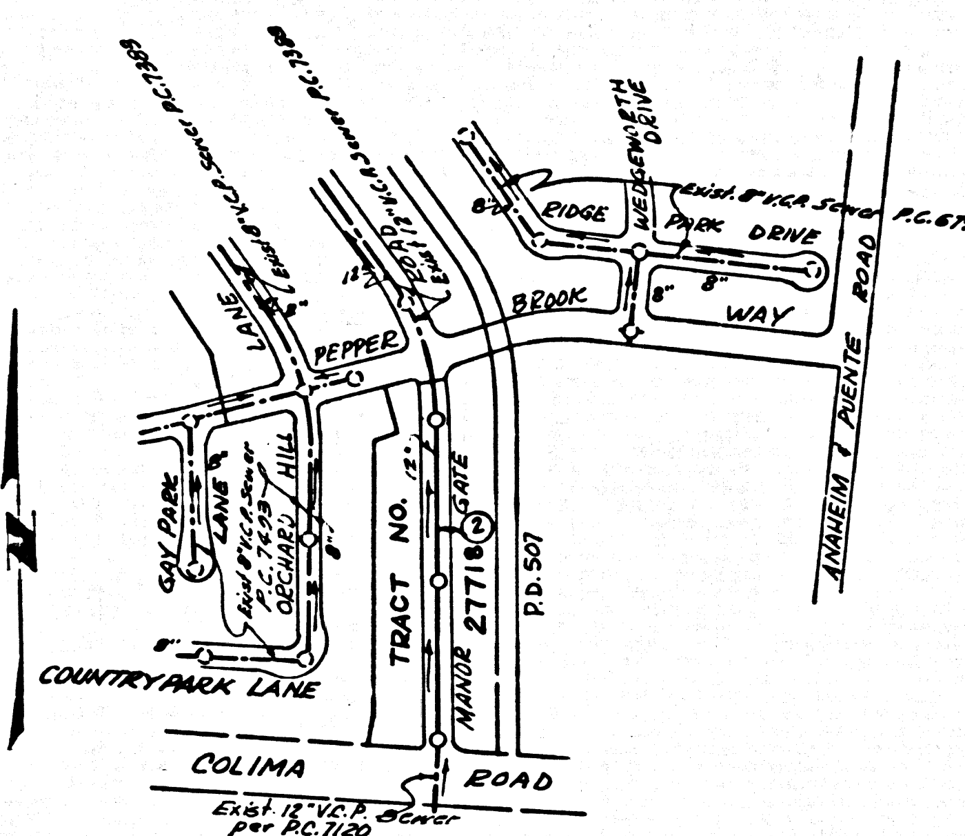
INDEX MAP - P.C. 7536 SCALE: 1" = 400'
